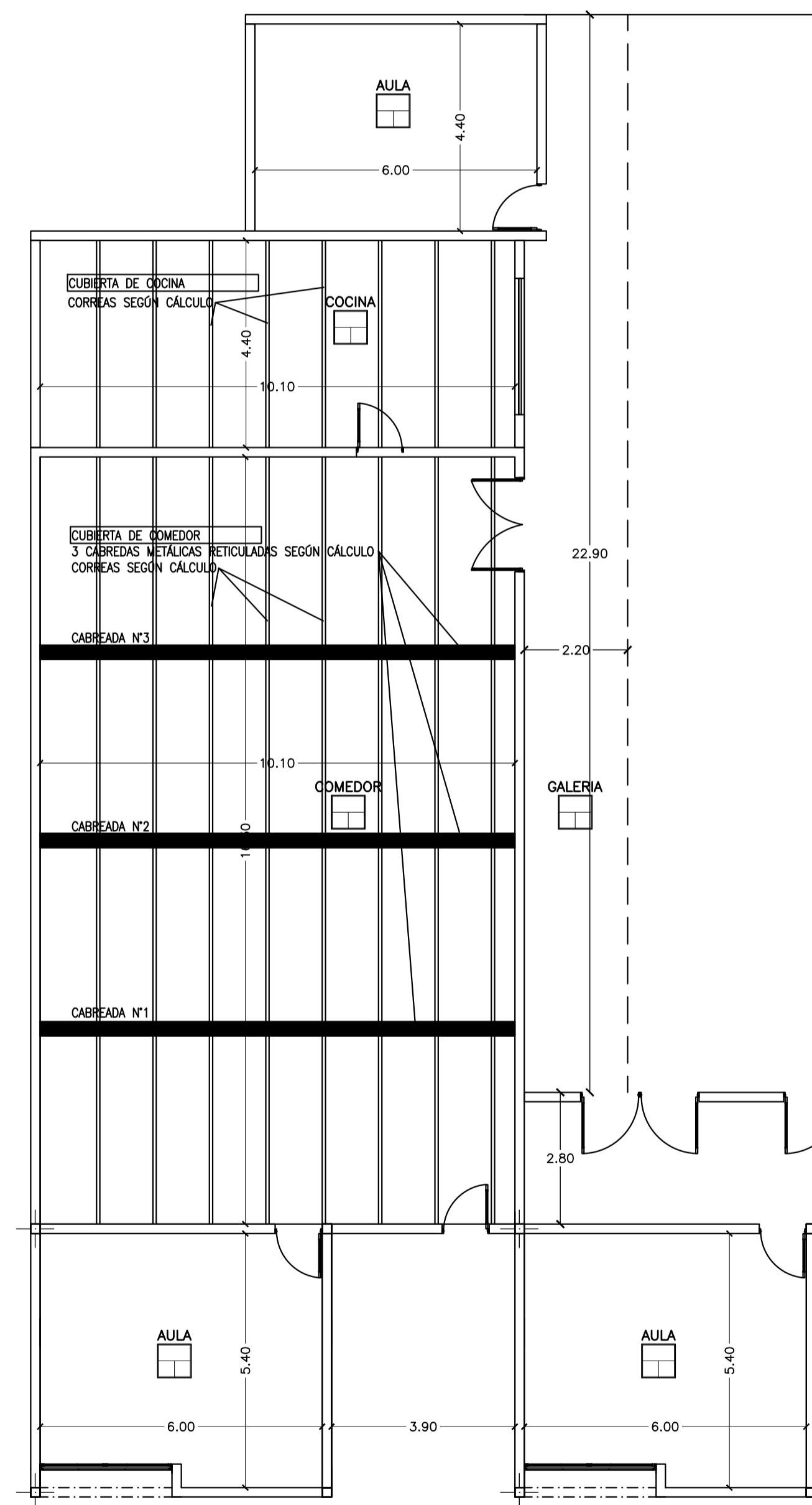
PLANTA BAJA
